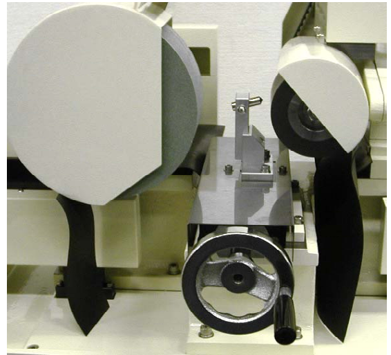
砥石車・調整車ツルーイング装置を装着したところ
