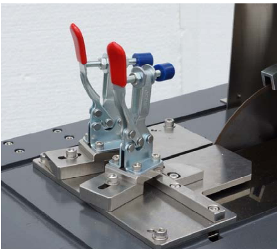
トグルクランプを開いたところ
