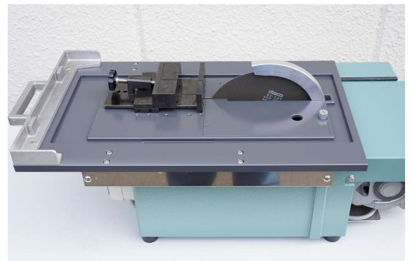
専用バイスダブルタイプを装着したところ
