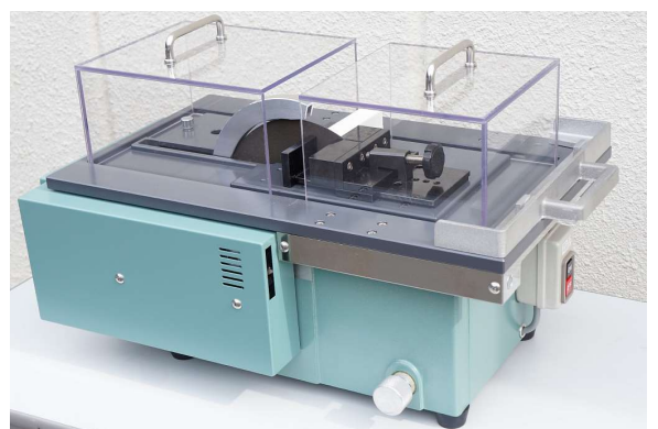
長尺試料加工時の前後カバー
