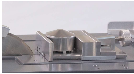
専用バイスダブルのクランプ例
